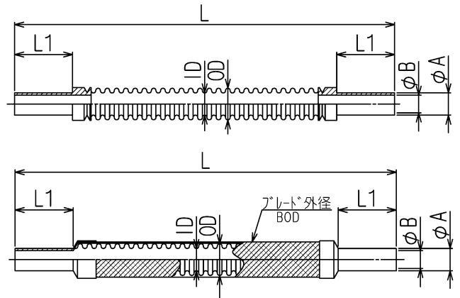
外観寸法図
