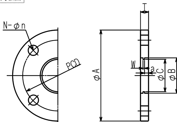
外観寸法図
