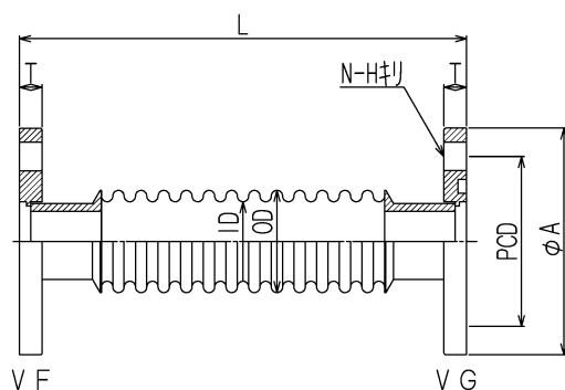
外観寸法図
