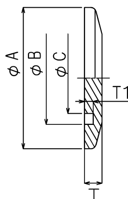
外觀寸法図
