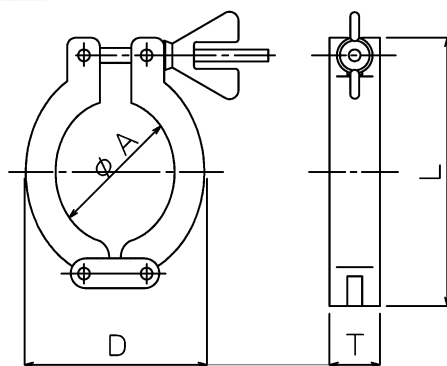
外観寸法図
