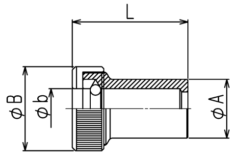
外観寸法図
