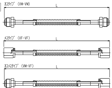
外観寸法図
