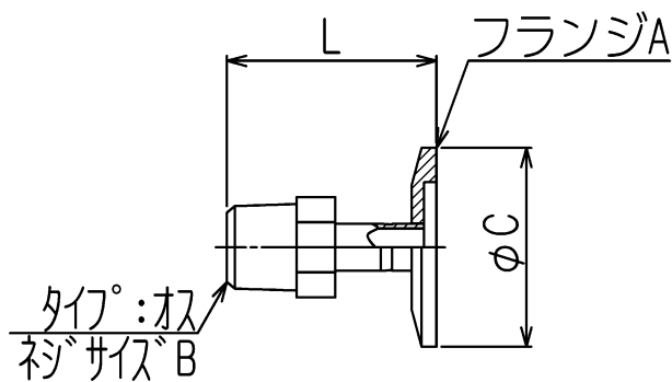
外觀寸法図
