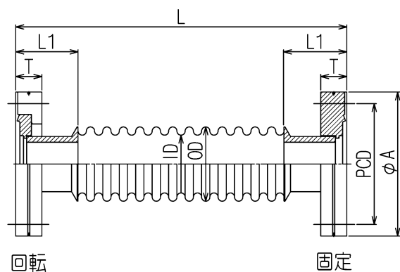
外観寸法図
