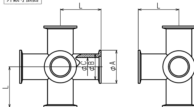
外観寸法図
