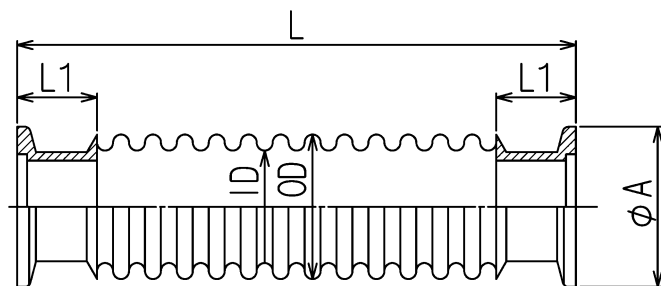
外観寸法図
