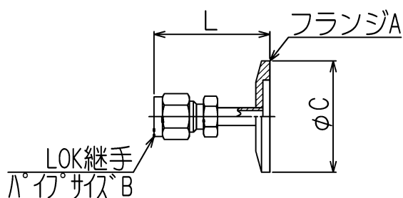
外観寸法図
