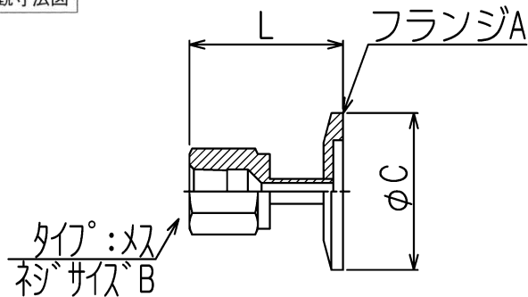
外觀寸法図
