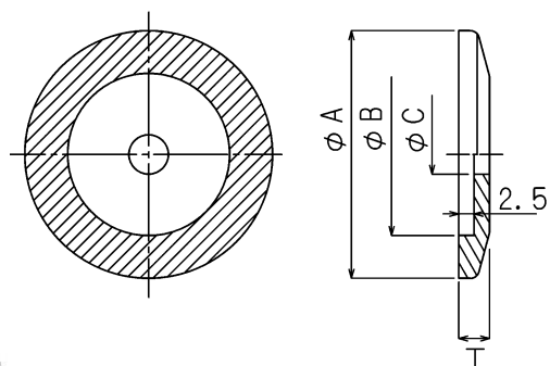
外観寸法図
