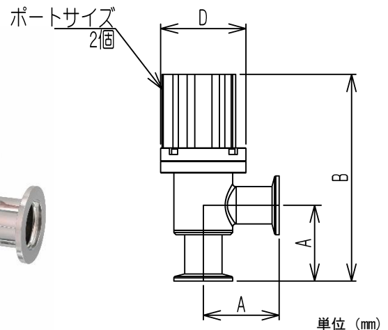
外観寸法図
