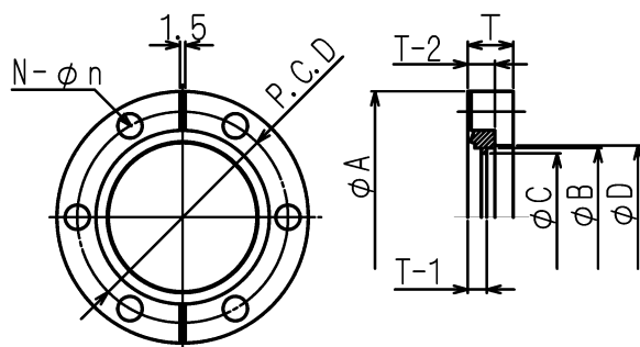
外観寸法図
