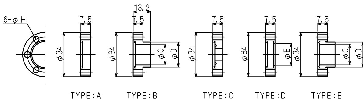
外観寸法図
