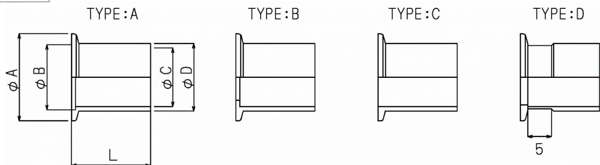
外観寸法図
