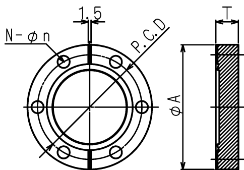
外観寸法図
