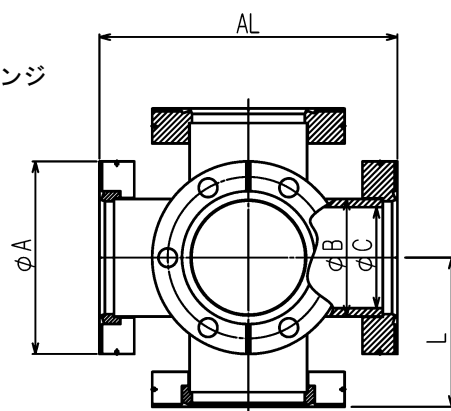
外観寸法図
