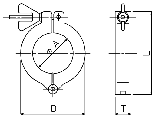
外観寸法図
