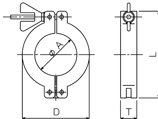
外観寸法図
