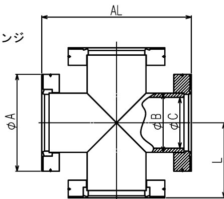
外観寸法図
